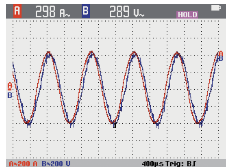
PM入力電流・電圧波形(参考)
